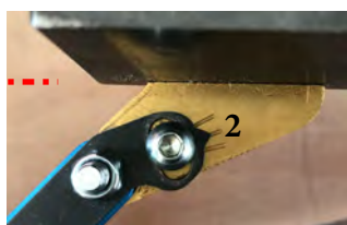
-Posizione sul carrello mobile del porta utensili della macchina. -Position on the tool post
